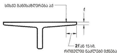
სურათი 721.2.2.1.2 ფილის სისქის განსაზღვრა დამრეცი სოფიტებისთვის
