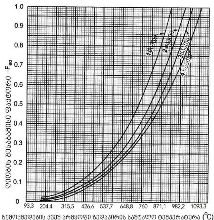
სურათი 705.7 ღიობის ეკვივალენტური ფაქტორი
