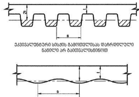
სურათი 722.2.2.1.3 ფილები დადარული ან ტალღოვანი სოფიტებით
